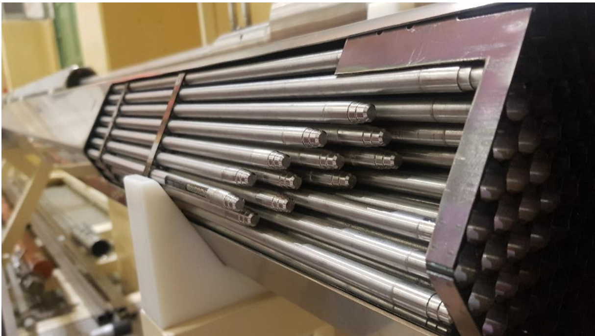
6. ábra – Fűtőkazetta
